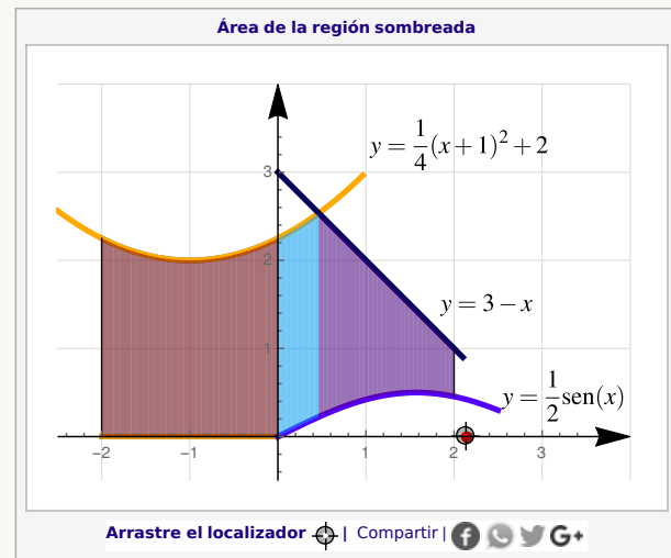
Figura 8.5: Región R = R_1 \cup R_2 \cup R_3
