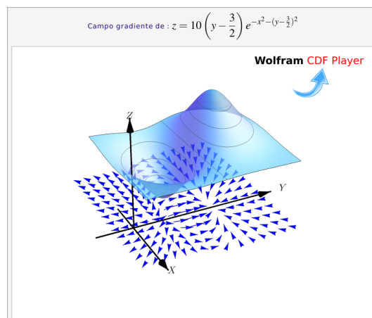
Figura 5.10: \nabla z(P) apunta en la dirección de máximo crecimiento respecto a cada punto P
