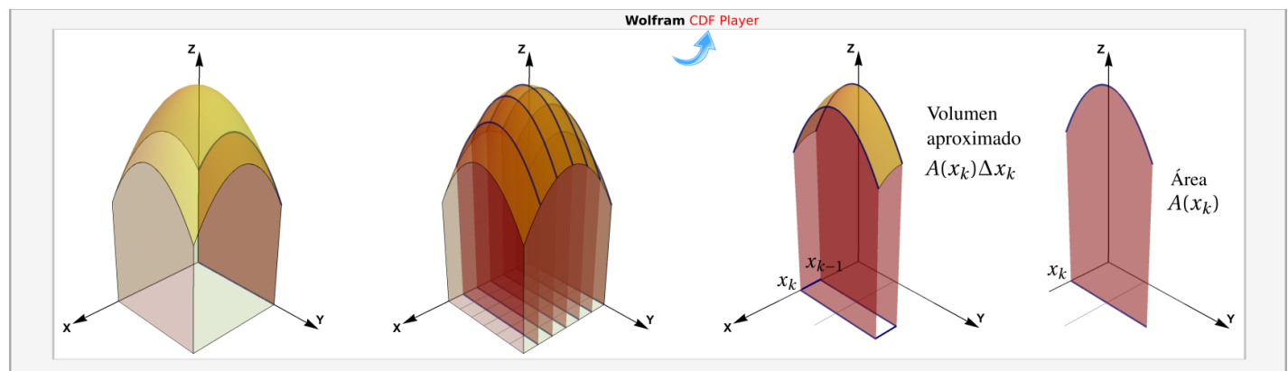
Figura 7.12: Volumen de Q aproximado como una suma del volúmenes de n rebanadas
