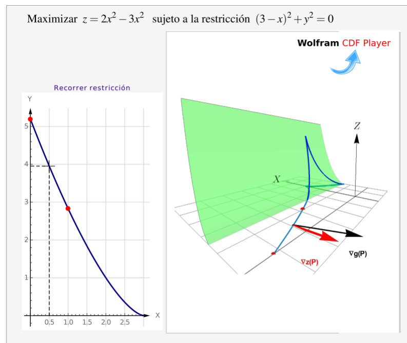
Figura 6.17: Máximo local se alcanza en (3,0) , pero éste no es punto crítico de L
