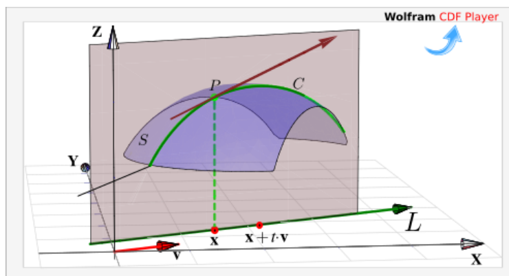
Figura 5.2: Derivada direccional en \mathbf{x} la dirección de \mathbf{v}
