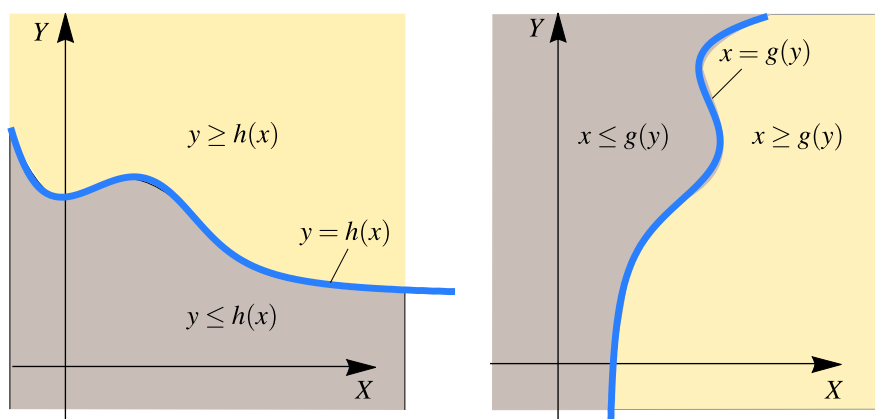
Figura 3.8: Representación de regiones definidas por desigualdades
