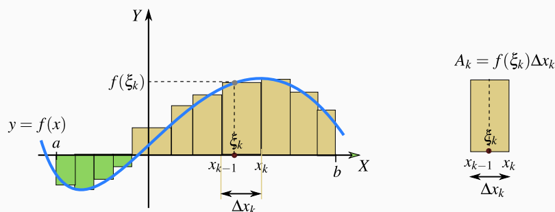
Figura 7.1: Suma de Riemann S_n (hacer clic para ver el widget)
