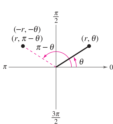
Figura 1.38: Simetría respecto a Eje Copolar
