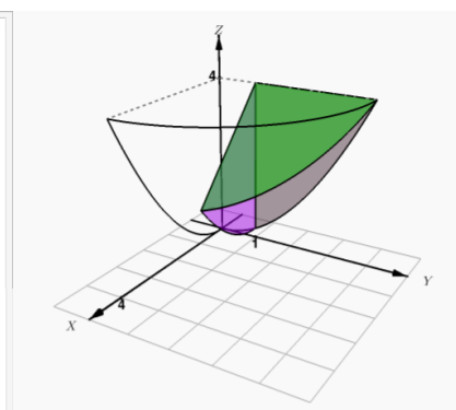
Figura 3.33: Sólido Q
