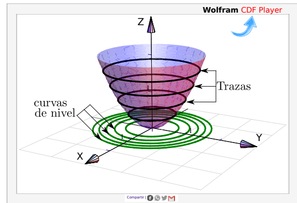
Figura 3.15: Algunas curvas de nivel y algunas trazas.
