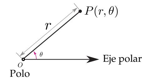
Figura 1.30: Coordenadas polares de P .
