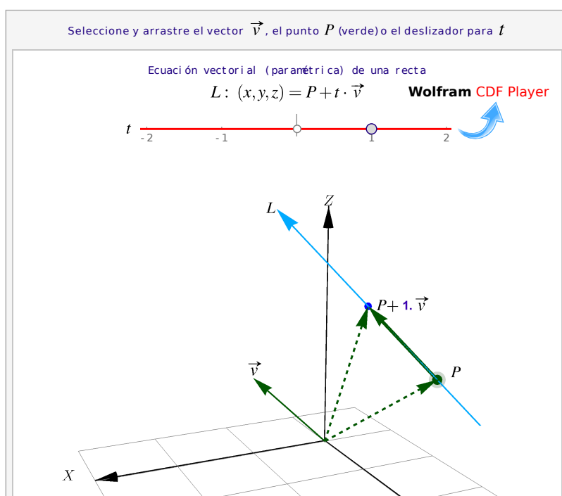
Figura 1.19: Ecuación vectorial de una recta
