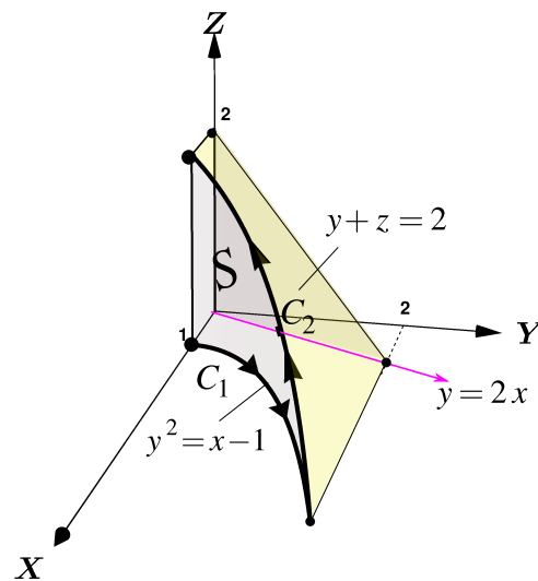
Figura 9.23: Curva C = C_1 + C_2 y superficie S
