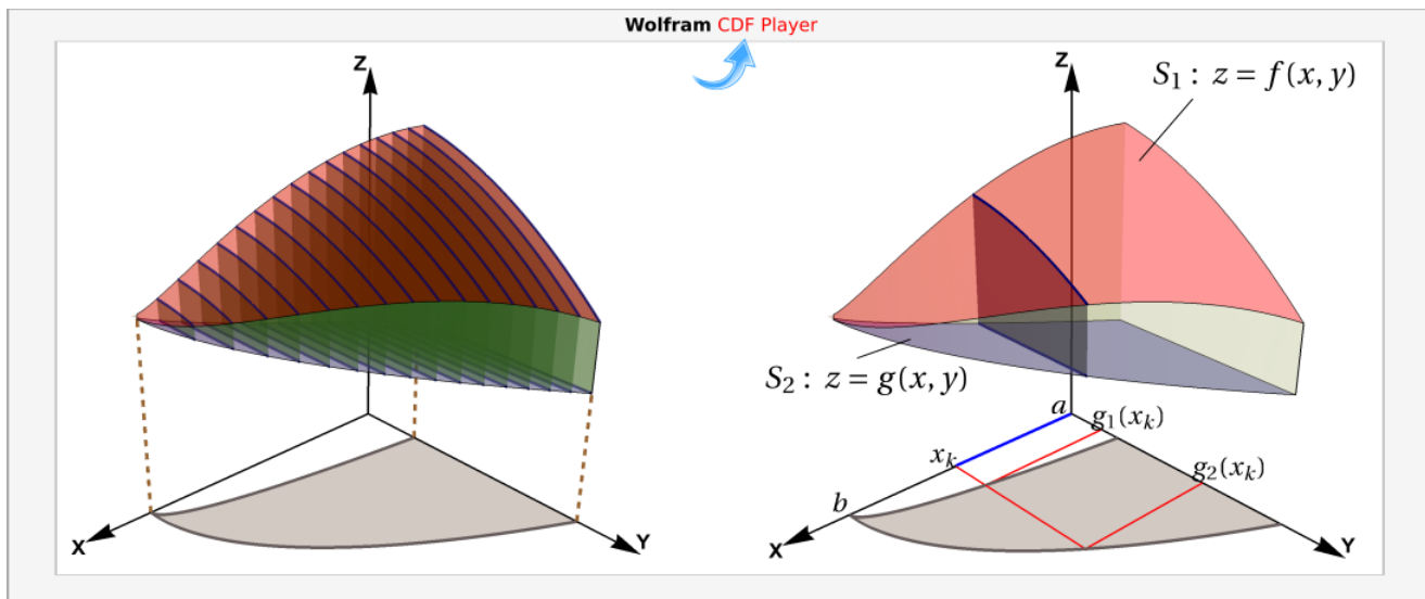
Figura 7.13: Cálculo de integral iterada, en el orden dydx
