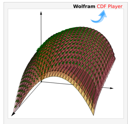
Figura 8.14: El flujo neto, por unidad de tiempo, es la suma de los flujos (volúmenes de los paralelepípedos)
