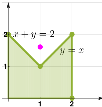
Figura 7.24: Centro de masa (\bar{x}, \bar{y})
