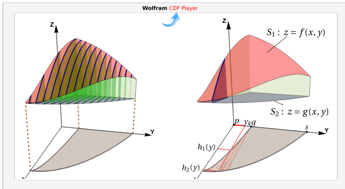
Figura 7.14: Cálculo de integral iterada, en el orden dx dy
