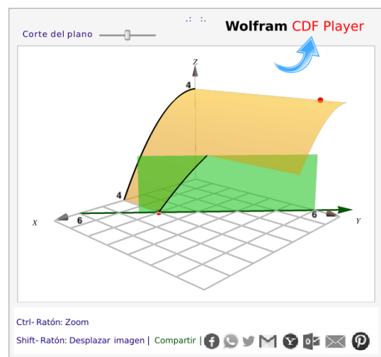
Figura 3.22: Curva de intersección entre las superficies S_1 : z = 4 - \frac{x^2}{4} y el plano S_2 : x + y = 6
