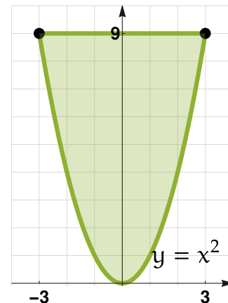
Figura 7.21: Región D : Lámina de densidad \rho(x, y) = x^2 + y .
