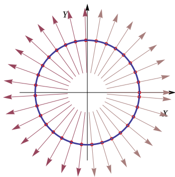
Figura 8.7: F_1 sobre x^2 + y^2 = 1 .
