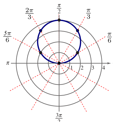
Figura 1.41: Gráfica de r = 4 \sin \theta
