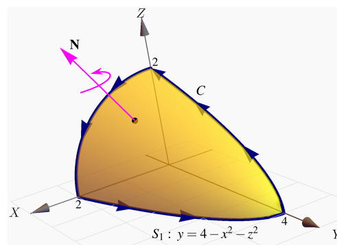
Figura 9.26: Curva C.
