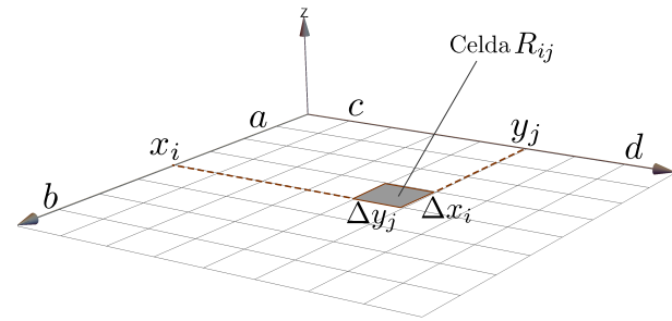
Figura 7.4: Malla de nm rectángulos
