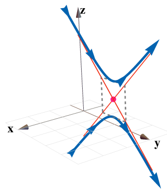
Figura 9.6: (z - 1)^2 - (y - 2)^2 = 1/2
