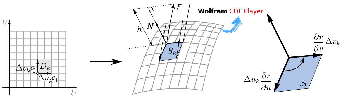
Figura 8.11: El fluido sobre S_k ocupa un paralelepípedo
