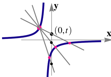
Figura A.3: Parametrización racional de \mathbf{C}
