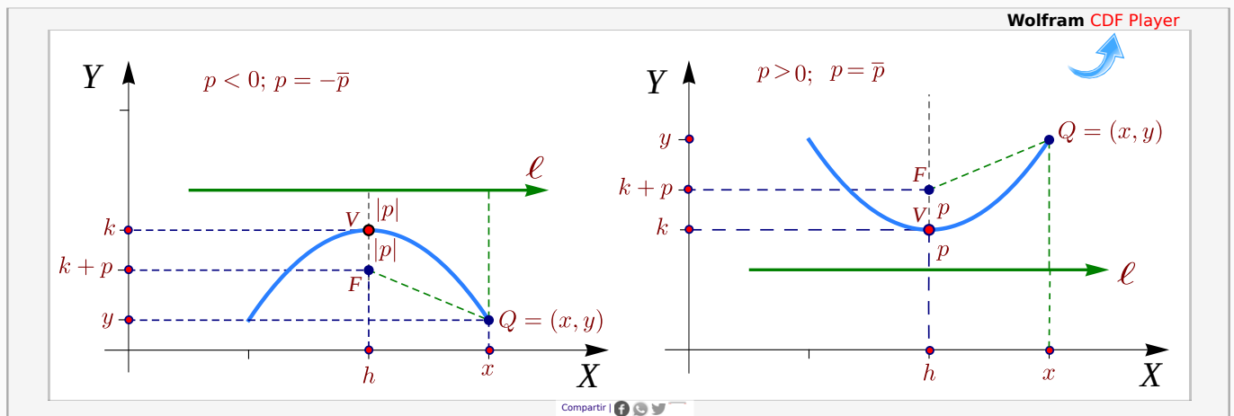
Figura 2.6: Parábola con directriz \ell : y = k - p , paralela al eje X.
