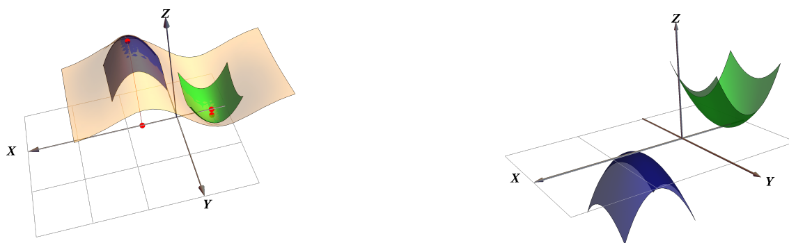
Figura 6.8: Polinomio de Taylor y las formas cuadráticas, con un solo signo!
