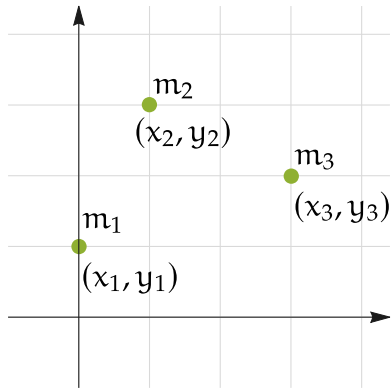
Figura 7.18: Sistema de k masas en \mathbb{R}^2
