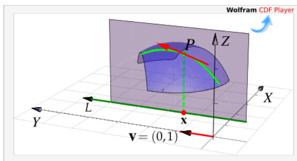
Figura 5.4: Derivada parcial en x en la dirección de Y
