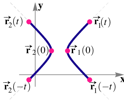
Figura 4.4: Simetría
