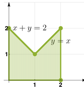
Figura 7.23: Lámina con \rho(x, y) = x + e^{5y+5}
