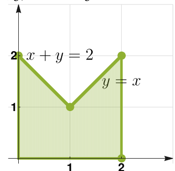
Figura 7.26: Lámina de densidad \rho(x, y) = x^2 + y^3
