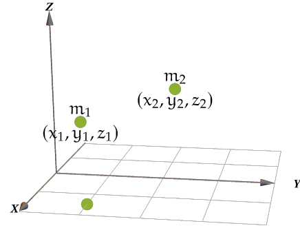
Figura 7.19: Sistema de k masas en \mathbb{R}^3
