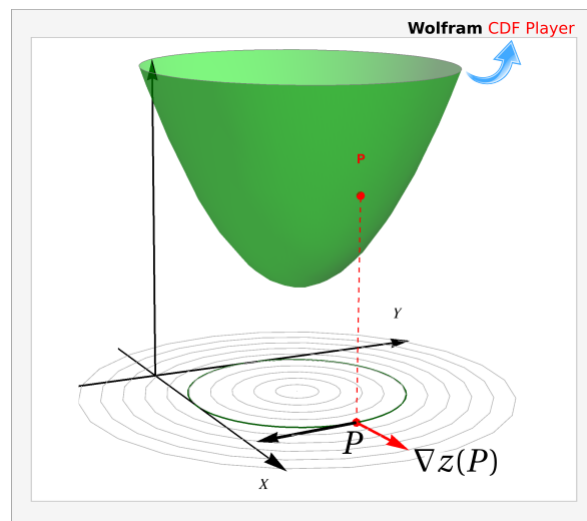
Figura 5.14: \nabla \mathbf{z}(x_0, y_0, z_0) es perpendicular a la curva de nivel z = z_0 .
