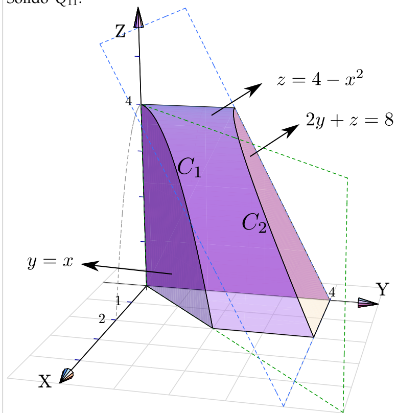
Sólido Q_{11} .
