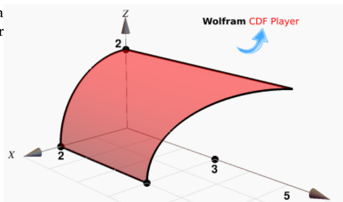
Figura 3.35: Superficie S_1 : x^2 + z^2 = 4
