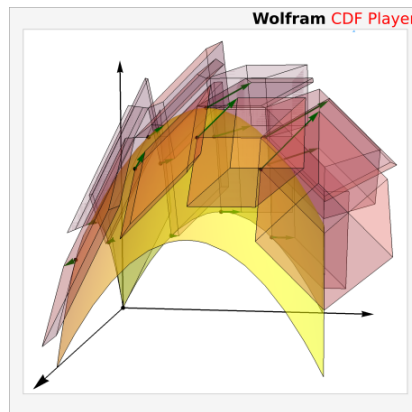
Figura 8.14: El flujo neto, por unidad de tiempo, es la suma de los flujos (volúmenes de los paralelepípedos)
