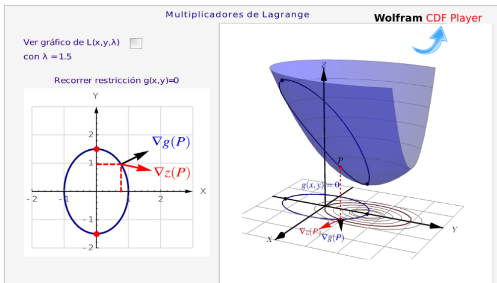
Figura 6.13: Un problema de optimización con restricciones.
