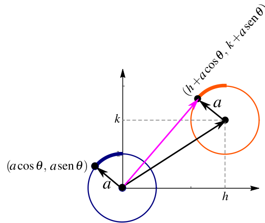
Figura 4.1: Una parametrización de la circunferencia
