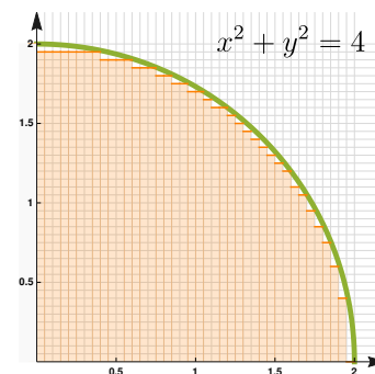
Figura 7.9: Malla con \Delta x = \Delta y = 0.05
