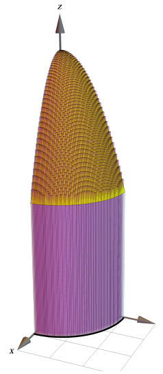
Figura 7.11: Malla con \Delta x = \Delta y = 0.05
