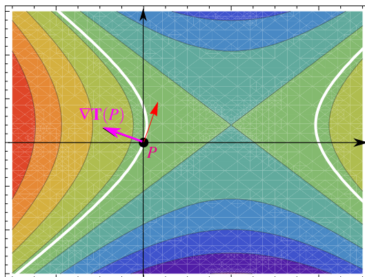
Figura 5.21: Mejor dirección, respecto a (0, 0) .
