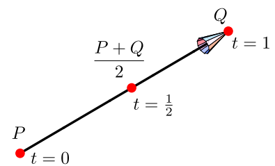
Figura 1.21: Punto medio
