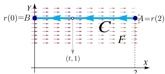
Figura 9.13: Curva C
