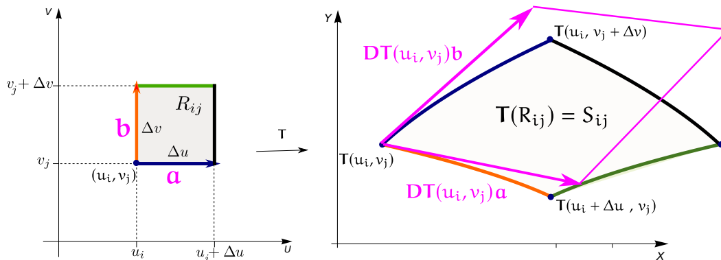
Figura 7.32
