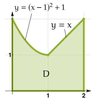
Figura 7.16: Región D
