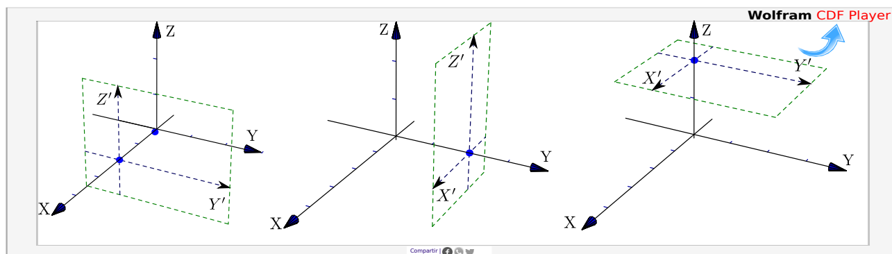
Figura 3.19: Traslación de ejes
