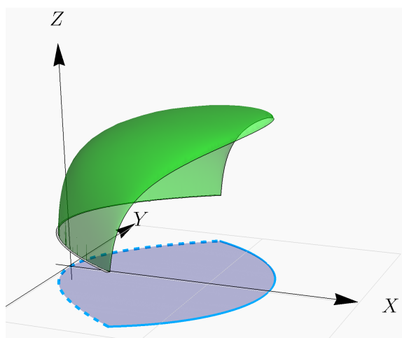
Figura 3.11: Superficie f(x, y) = \ln(x - y^2) + \sqrt{1 - y^2 - \frac{x^2}{2}} y su dominio
