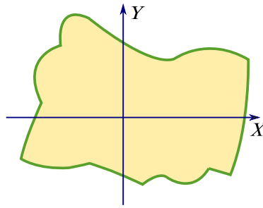
Figura 7.20: “Lámina” D con densidad \rho(x, y) en cada punto (x, y)
