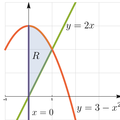
Figura 7.15: Región de integración R
