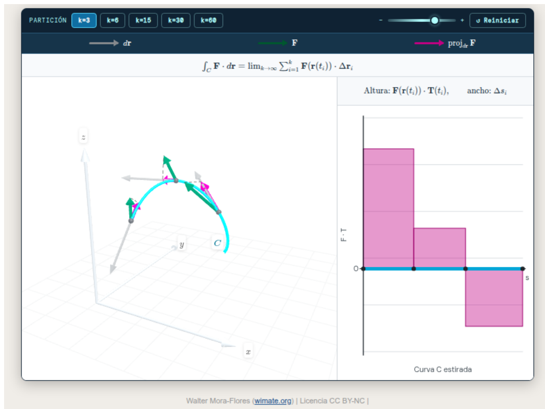
Figura 9.11
