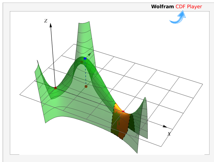
Figura 6.11: f(x, y) = 6xy - 2x^2y - 3xy^2
