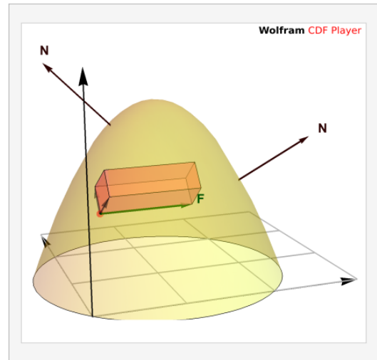
Figura 8.13: El fluido sobre S_k en contra la “dirección” de \mathbf{N}
