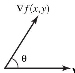
Figura 5.20
