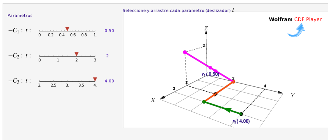
Figura 9.7: Curva C = C_1 + C_2 + C_3
