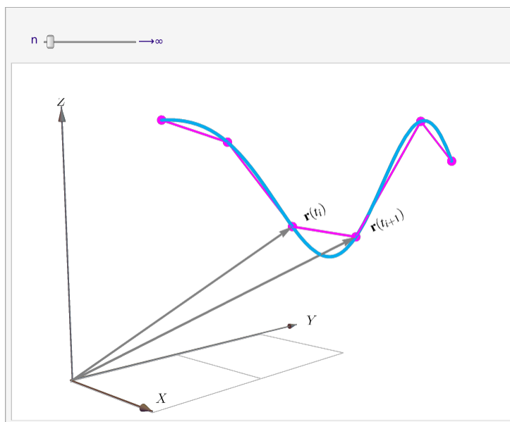
Figura 9.8: Longitud de arco como una integral de Riemann.
