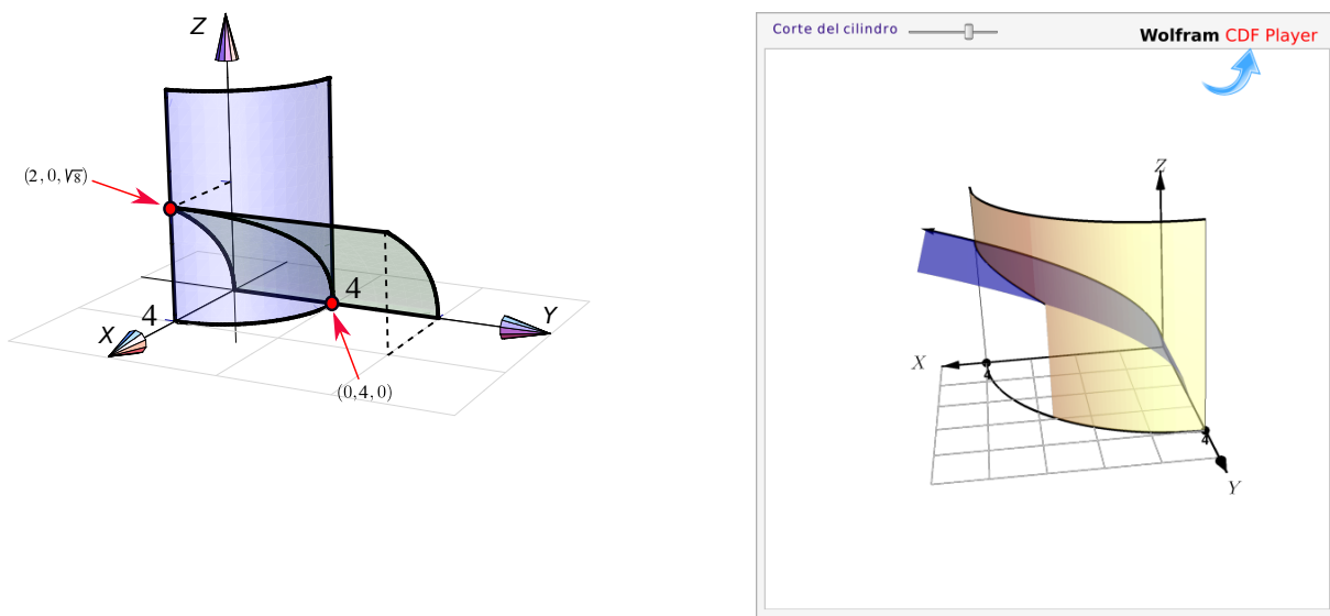
Figura 3.25: Curva de intersección las superficies S_1 : x^2 + y^2 = 16 y S_2 : 2x - z^2 = 0
