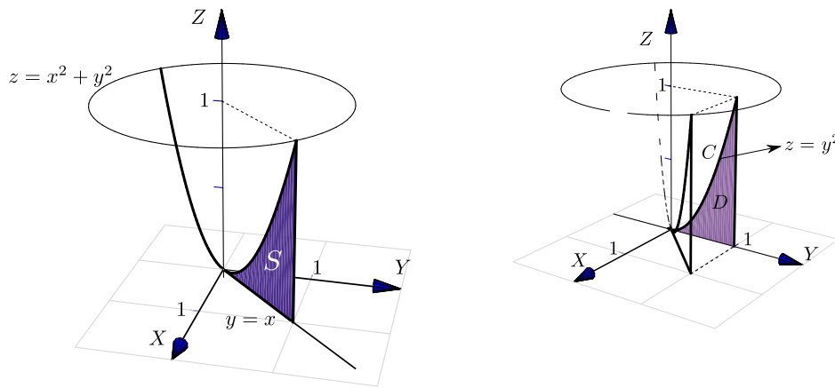
Figura 8.16: Superficie S
