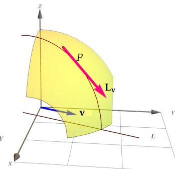
Figura 5.24: \mathbf{v} = (v_0, v_1)
