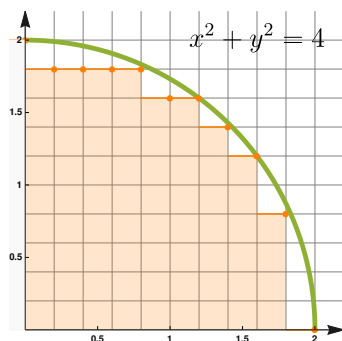
Figura 7.8: Malla con \Delta x = \Delta y = 0.2
