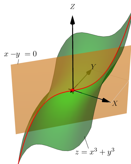
Figura 6.14: (0, 0, 0) es punto crítico de L pero no es solución del problema
