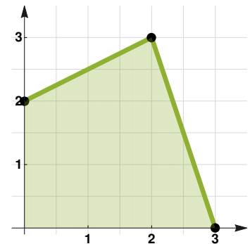
Figura 7.25: Lámina de densidad \rho(x, y) = 3x^2 + 3y^2
