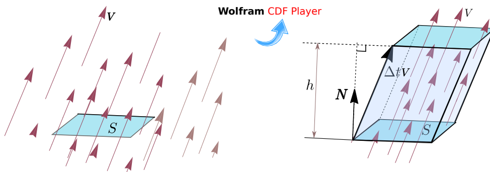
Figura 8.10: El fluido sobre S llena un paralelepípedo
