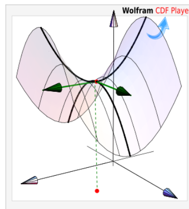
Figura 6.5: En los puntos de silla, \nabla f(\mathbf{p}) = 0
