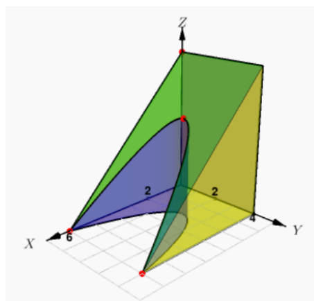
Figura 3.31: Sólido Q
