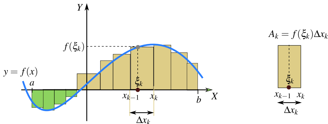
Figura 7.3: Suma de Riemann S_n (hacer clic para ver el widget)
