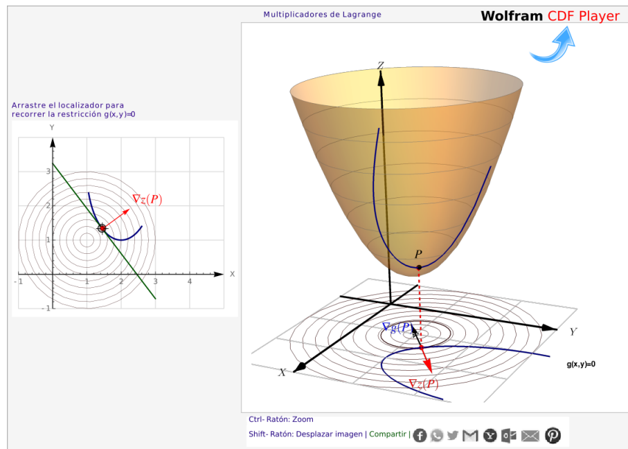
Figura 6.12: Un problema de optimización con restricciones.
