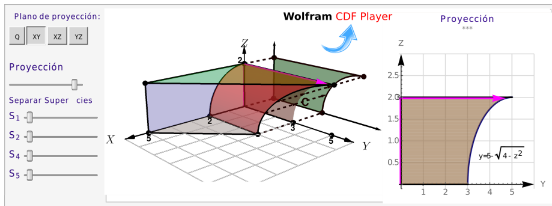
Figura 3.41: Proyección del sólido Q sobre el plano YZ
