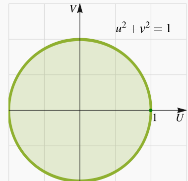
Figura 7.29: Superficie S
