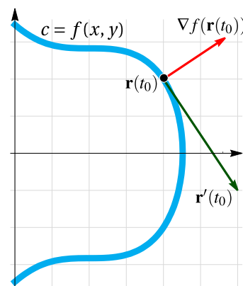
Figura 5.13: El gradiente es perpendicular a las curvas de nivel
