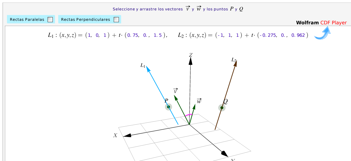
Figura 1.22: Ángulo, paralelismo y perpendicularidad
