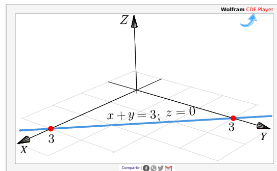
Figura 3.13: Recta x + y = 3 en el espacio tridimensional
