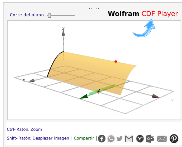
Figura 3.21: Curva de intersección entre las superficies S_1 : z = 1 - x^2 y el plano S_2 : y = 3
