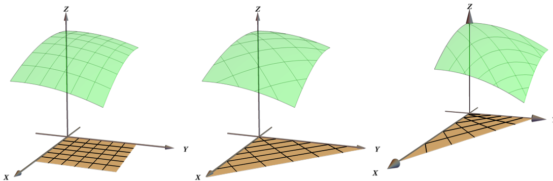
Figura 7.30: Una misma función con distintas regiones de integración que requieren distintos cambios de variable
