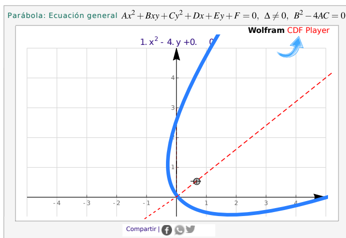
Figura 2.3: Parábola con rotación: B \neq 0
