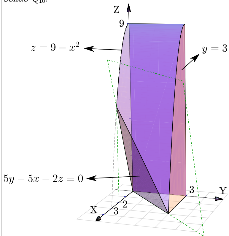
Sólido Q_{10} .
