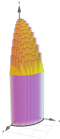
Figura 7.10: Malla con \Delta x = \Delta y = 0.2
