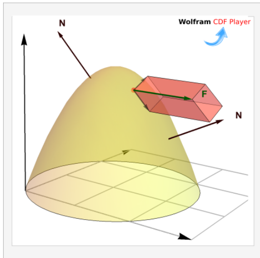
Figura 8.12: El fluido sobre S_k en “dirección” de \mathbf{N}
