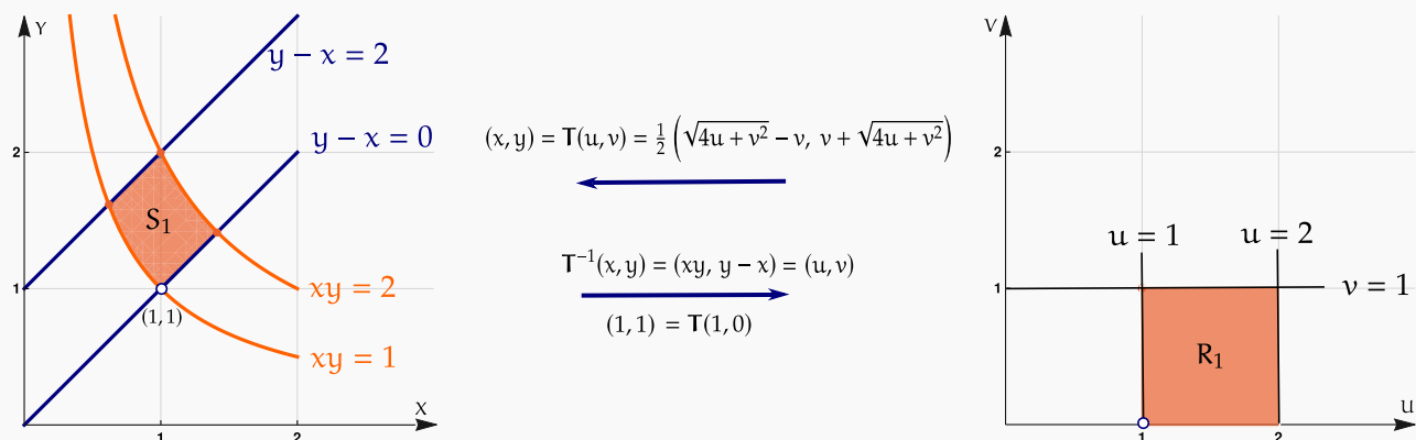
Figura 7.27: Cambio de variable (u, v) = T^{-1}(x, y)
