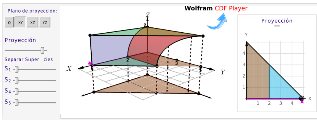
Figura 3.40: Proyección del sólido Q sobre el plano XY
