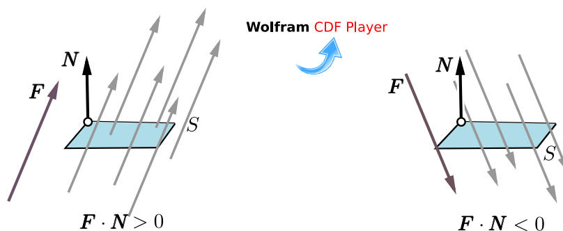
Figura 8.15: S se orienta con \mathbf{N} . \iint_S \mathbf{F} \cdot \mathbf{N} \, dS calcula el flujo neto en “la dirección” del \mathbf{N} escogido
