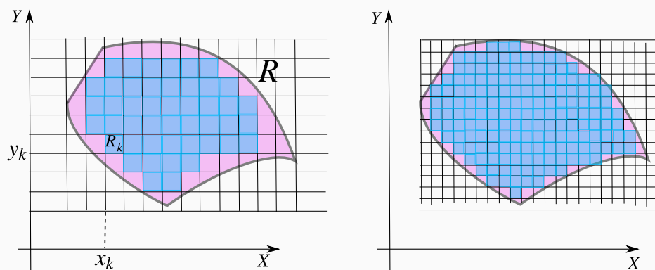
Figura 7.7
