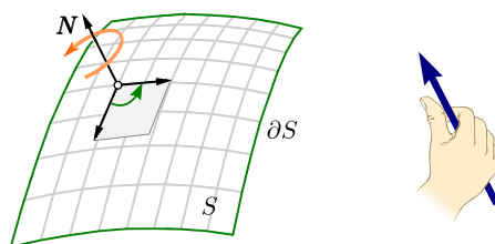
Figura 9.25: Orientación positiva de C respecto a \mathbf{N} .
