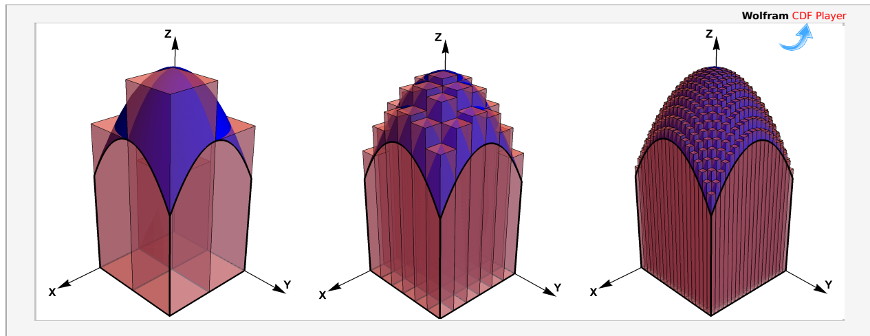
Figura 7.6: Aproximación del volumen de un sólido con sumas de Riemann
