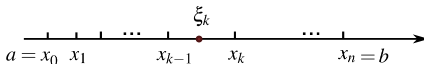
Figura 7.2: Partición de [a, b]
