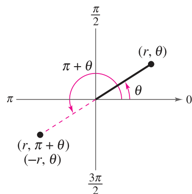
Figura 1.39: Simetría respecto al Polo
