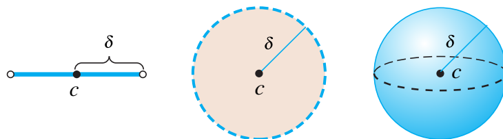
Figura 5.1: Entornos abiertos alrededor de c y de radio \delta , en \mathbb{R} , \mathbb{R}^2 y \mathbb{R}^3 (con la distancia euclidiana)
