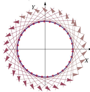
Figura 8.8: F_2 sobre x^2 + y^2 = 1 .
