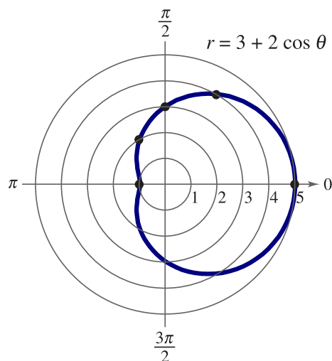
Figura 1.40: La curva r = 3 + 2 \cos \theta presenta simetría respecto al Eje Polar
