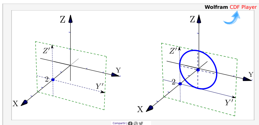
Figura 3.20: Traslación de ejes y dibujo de la traza x = 2
