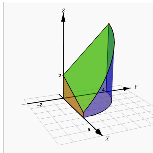
Figura 3.32: Sólido Q
