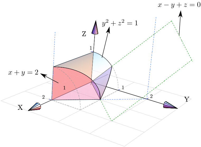
Sólido Q_3 .
