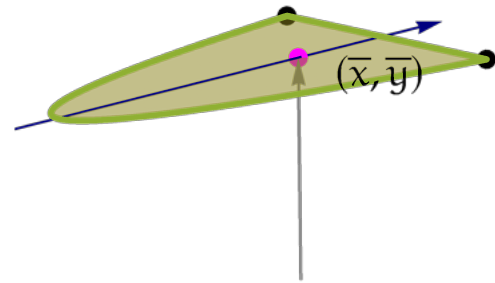
Figura 7.22: Centro de masa (\bar{x}, \bar{y})
