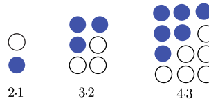
Figura 1.6. 2t_1 = 2 \cdot 1 , 2t_2 = 3 \cdot 2 , 2t_3 = 4 \cdot 3, \dots
