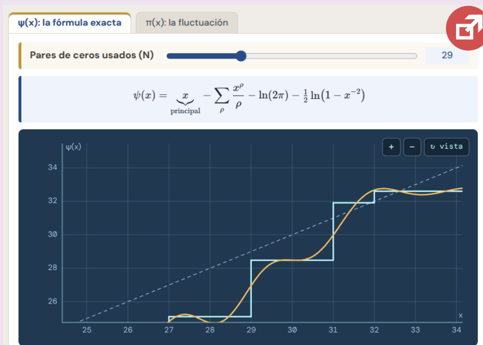
Figura 7.1. Ceros de \zeta y conteo de primos
