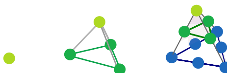
Figura 1.9. T_1 = 1 , T_2 = 4 , T_3 = 10 ,...
