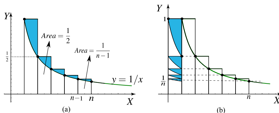
Figura 7.2. Comparando el área \ln(n) con la suma H_n .
