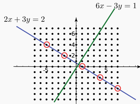
Figura 2.2. Algunas soluciones enteras de la ecuación 2x + 3y = 2 .
