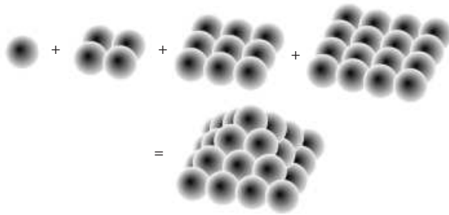
Figura 1.12. P_4 = 30
